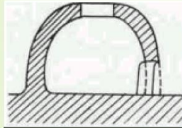
Домна из Лабенского городища (разрез)
