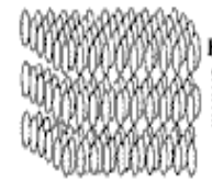
Смектическая фаза
